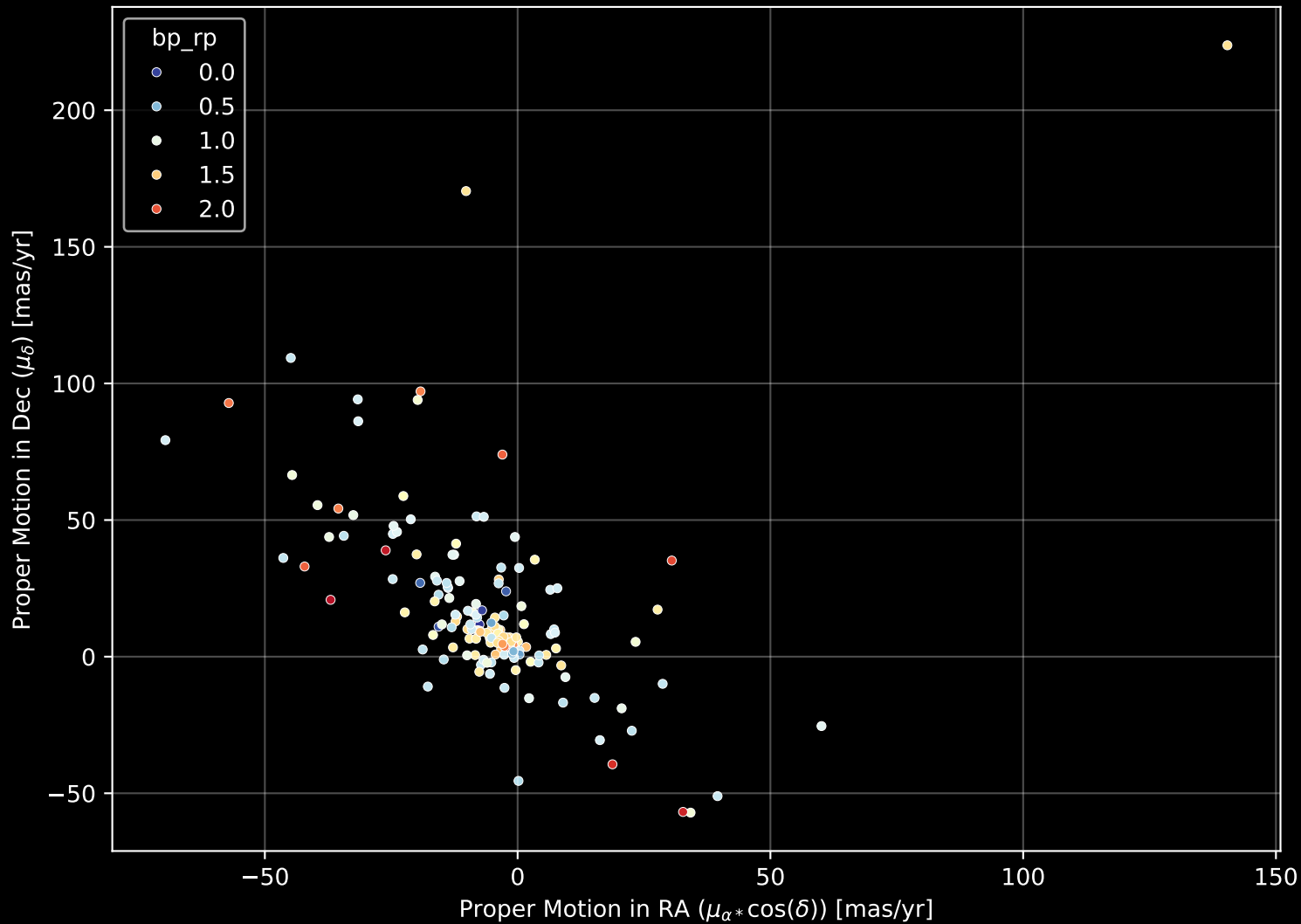
APOGEE DR17 Field: [283-19-O_TESS] Proper Motion Diagram (n= 161)
