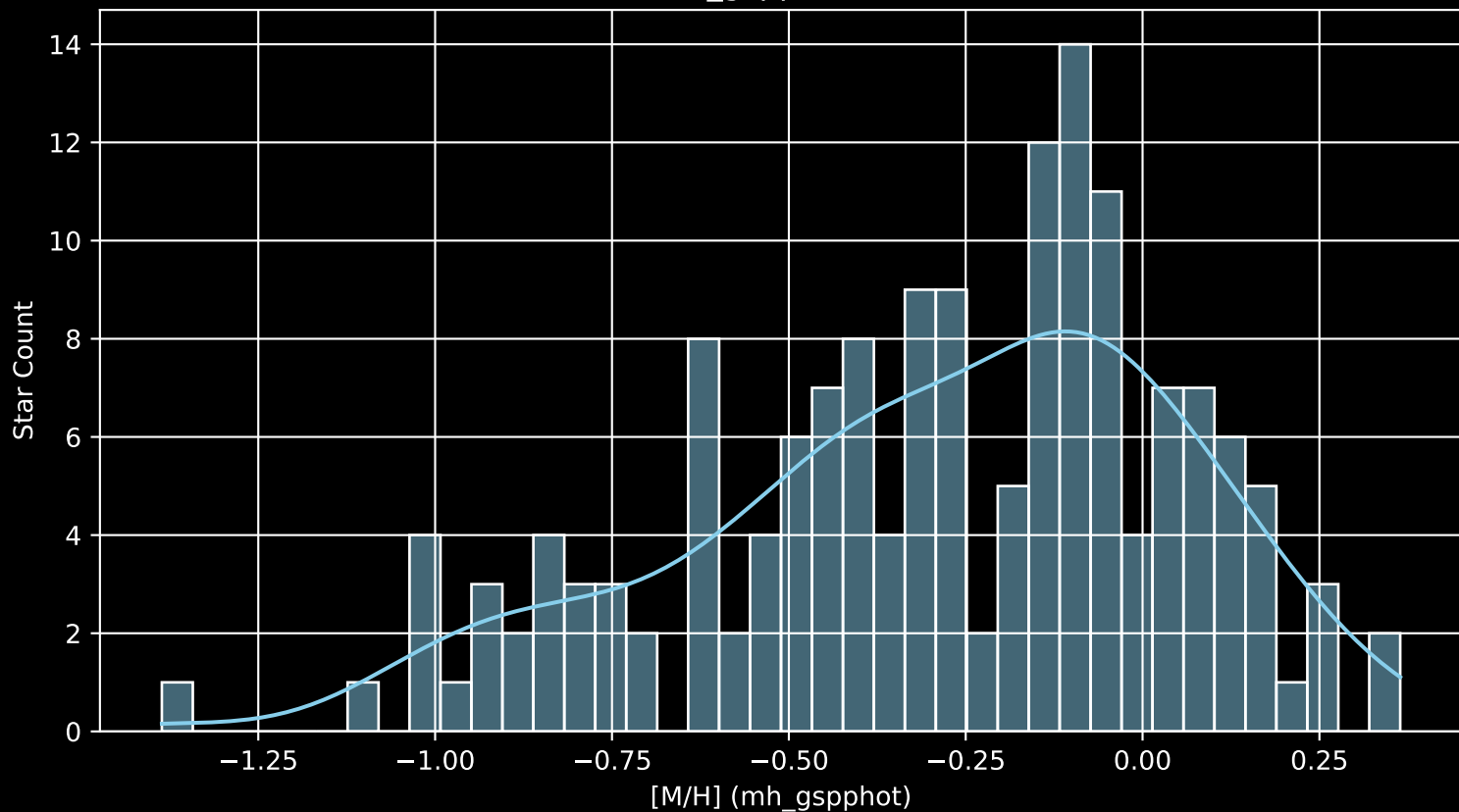
APOGEE DR17 Field: [283-19-O_TESS [M/H] (mh_gspphot) (n= 160)
