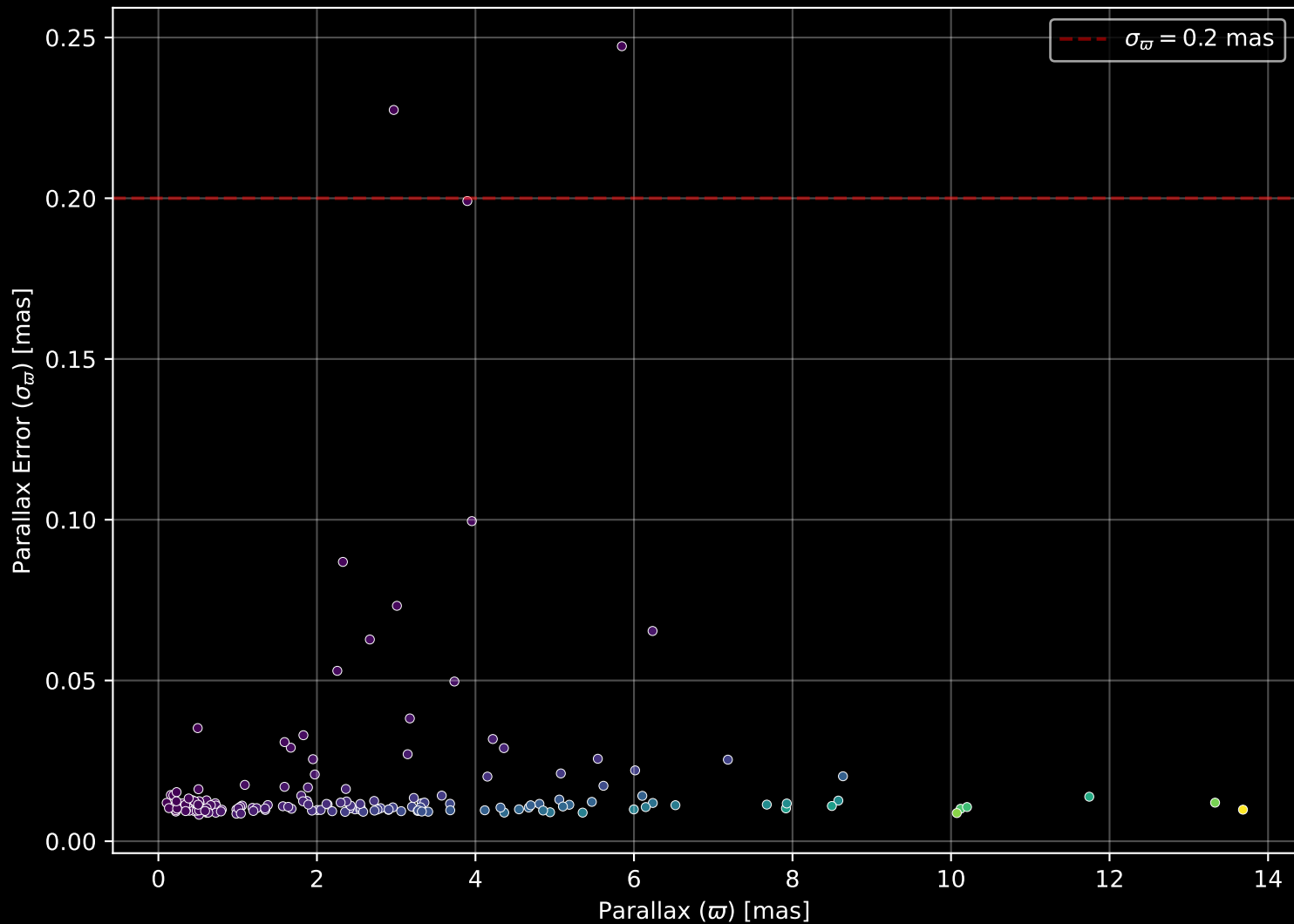
APOGEE DR17 Field: [283-19-O_TESS] Parallax Quality (n= 161)
