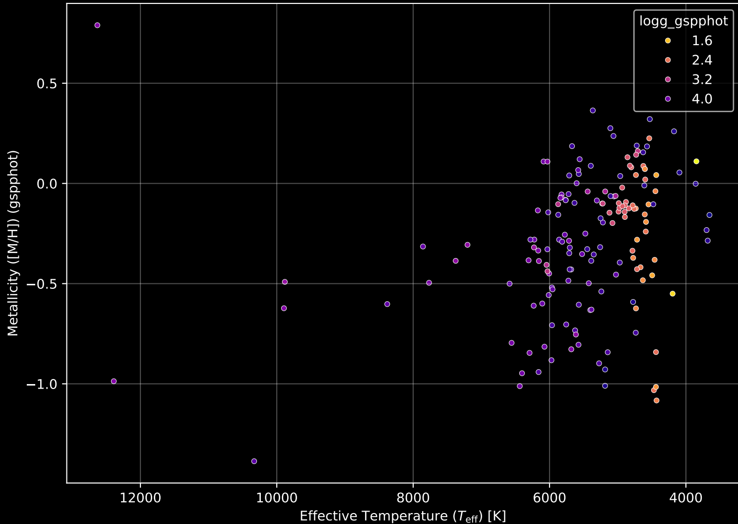
APOGEE DR17 Field: [283-19-O_TESS] Stellar Population Parameters (n= 161)
